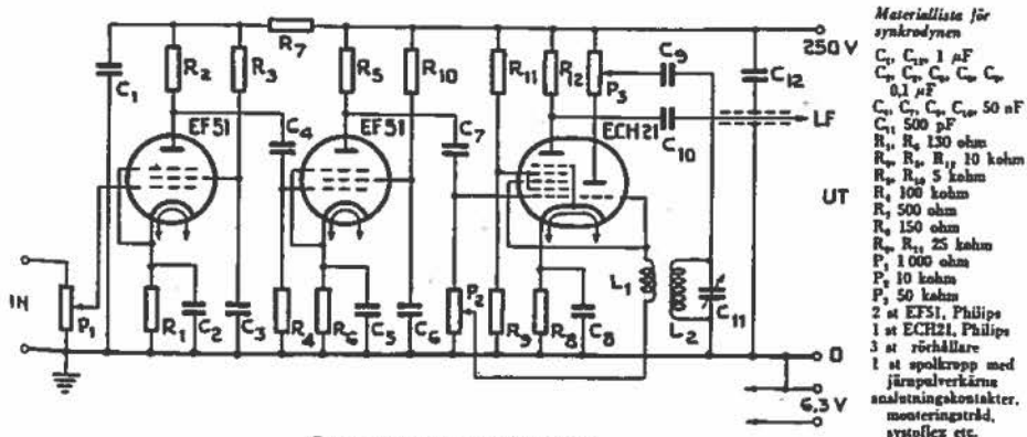
Fig. 1. Synkrodynens kopplingschema.
